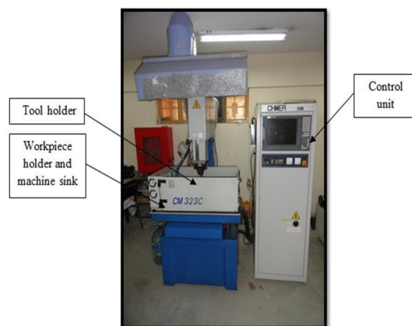
Fig.2 : EDM CM323C machine.
