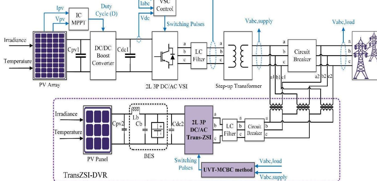
FigureB:PVfedZSI-DVRConfiguration
