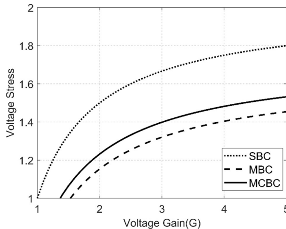
Fig:DifferentcontrolmethodsinZSI
