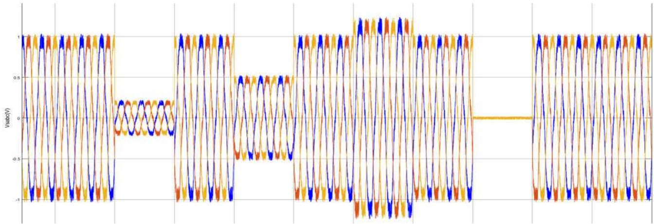
Fig:Supplyvoltage
