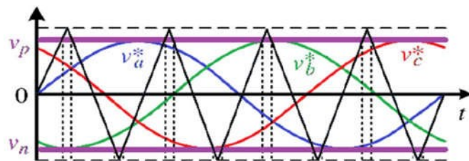
FigA:SBCMethod
