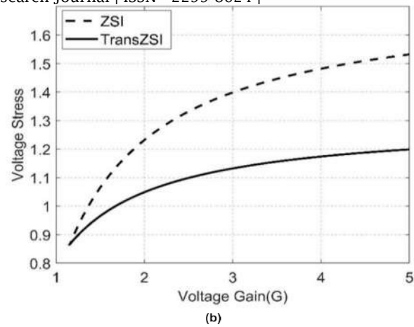
Fig:MCBCMethodinZSIandTRANS-ZSI
